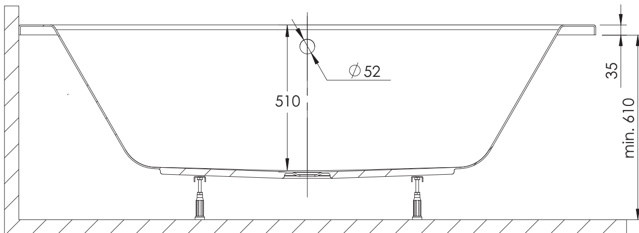
PRZEKRÓJ A-A
