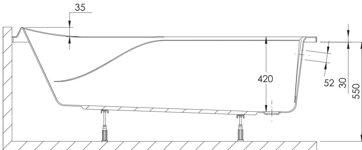
PRZEKRÓJ A-A
