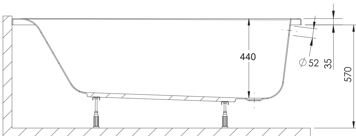
PRZEKRÓJ A-A
